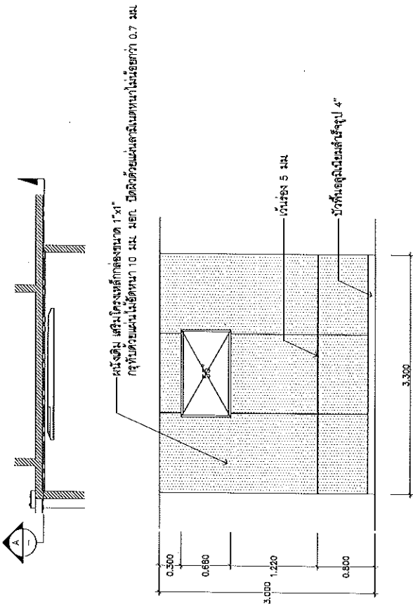
ELEVATION - E (ห้องอ่านวารสาร) SCALE 1:50
